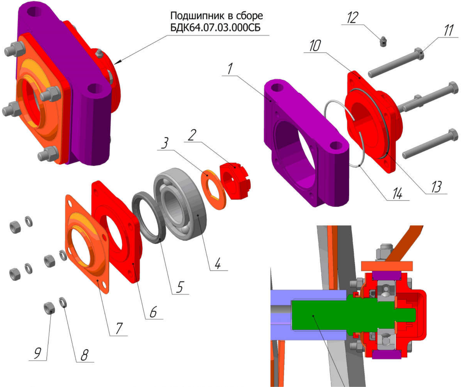
Подшипник катка в сборе БДК64.07.03.000СБ
